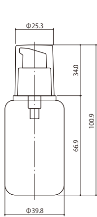
HB030-RO/UL-A
