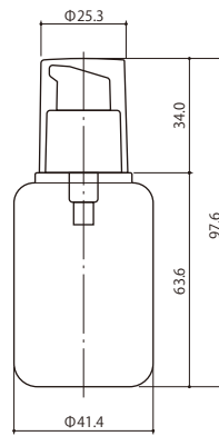
HB035-RO/UL-A
